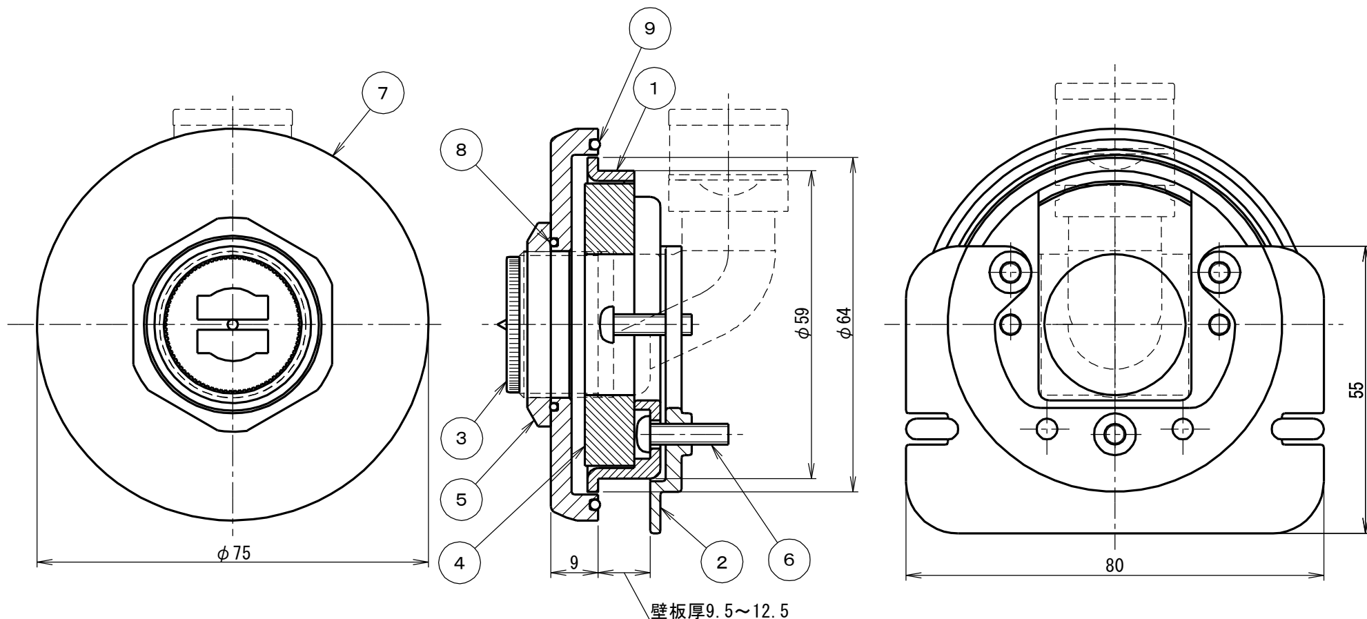
製品仕様図
